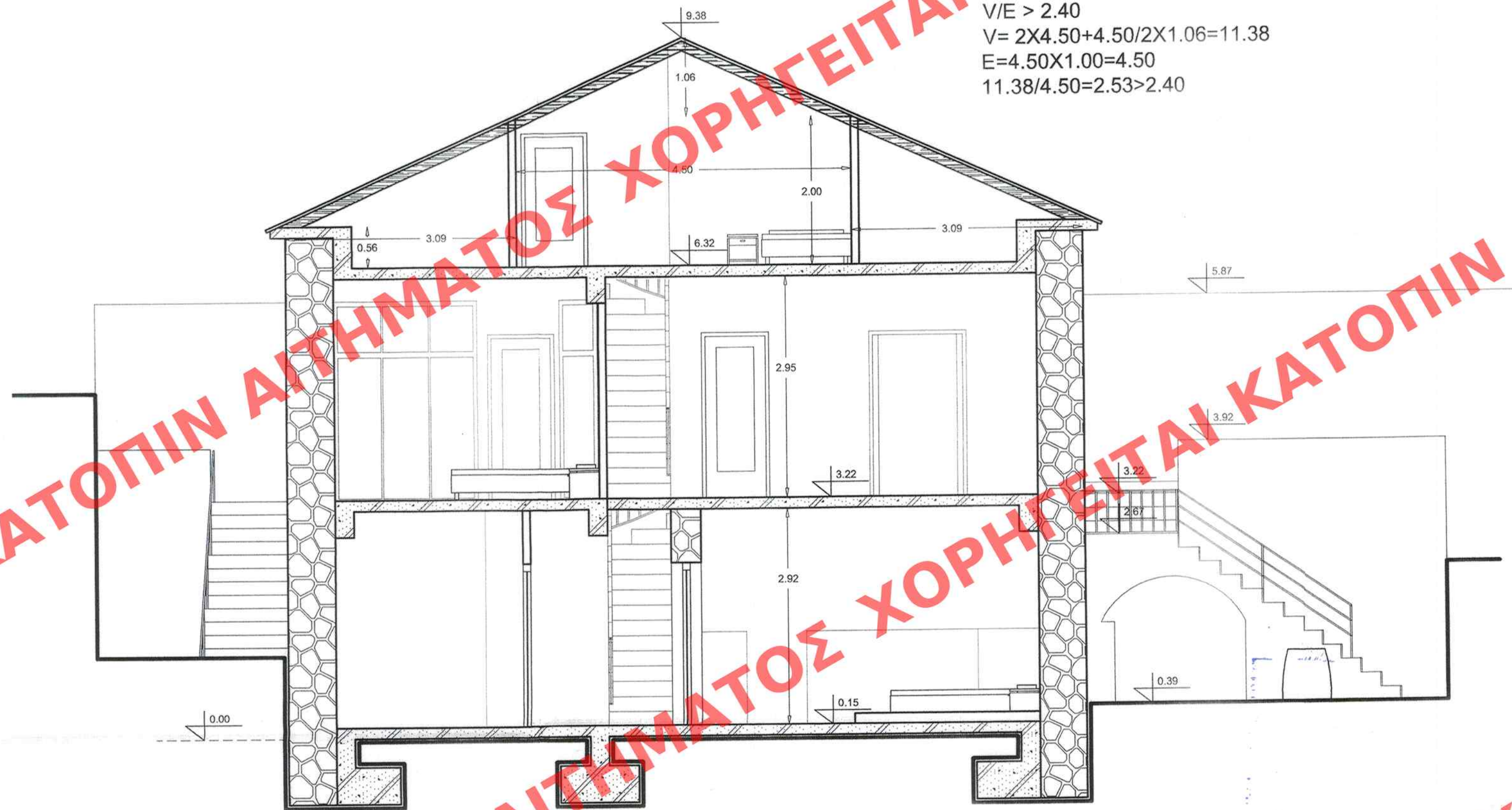
TOMH B-B
